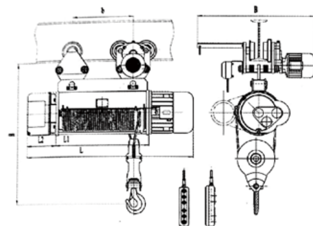
CD 1 /MD 1 型 0.5-5吨 (H=12-30米) Model CD 1 /MD 1 0.5-5T (H=12-30m)
