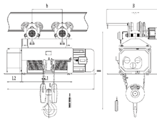
HY II型 10吨 (H=9-20米) Model HY II 10T (H=9-20m)
