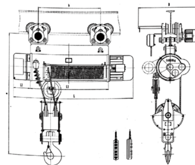
CD 1 /MD 1 型 16吨 (H=9-30米) Model CD 1 /MD 1 16T (H=9-30m)
