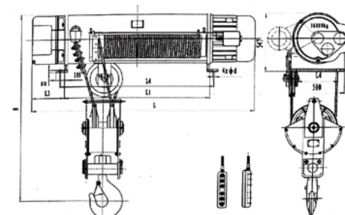
CD 1 /MD 1 型固定式 16吨 (H=9-30米) Model CD 1 /MD 1 Stationary 16T (H=9-30m)
