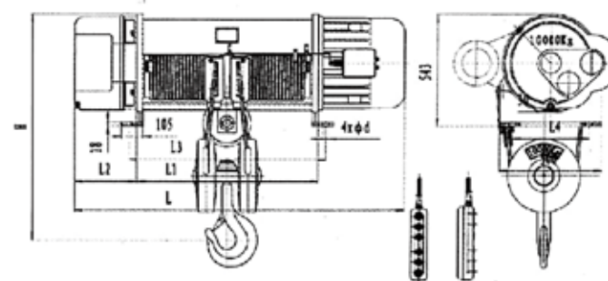
CD 1 /MD 1 型固定式 10吨 (H=9-30米) Model CD 1 /MD 1 Stationary 10T (H=9-30m)
